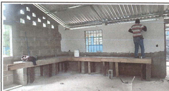
Foto 4: Remozamiento de paredes de interior de cocina.
